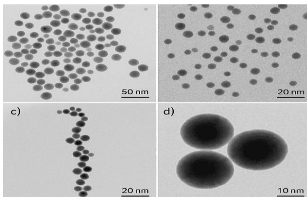
Figure 5: TEM images
