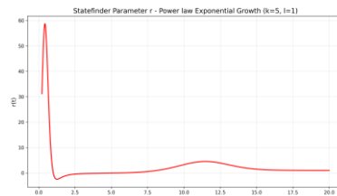
(a) Statefinder parameter r(t)
