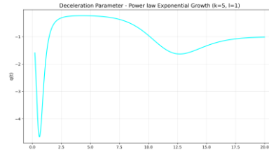
(b) Deceleration parameter
