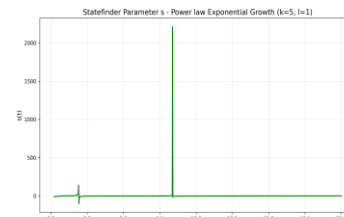
(b) Statefinder parameter s(t)
