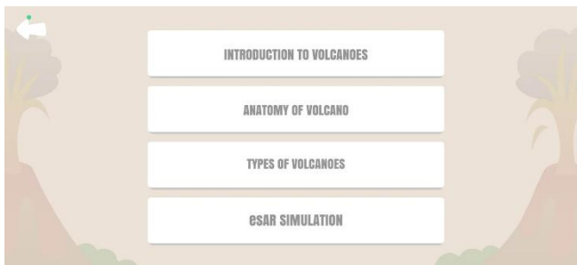
Fig. 4 EsAR Menu
