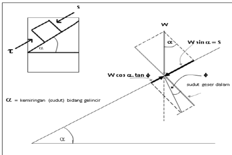
Gambar 2.1 Gaya yang Bekerja Pada Lereng
