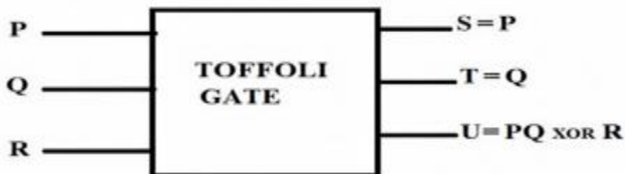
Fig. 3.4. Toffoli Gate
