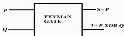
Fig. 3.2. Feynman Gate
