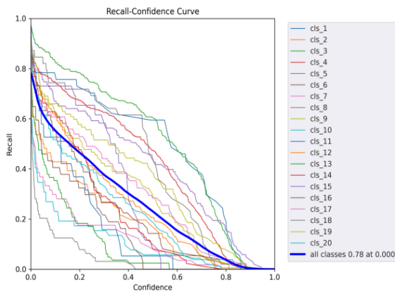
YOLOv5s
