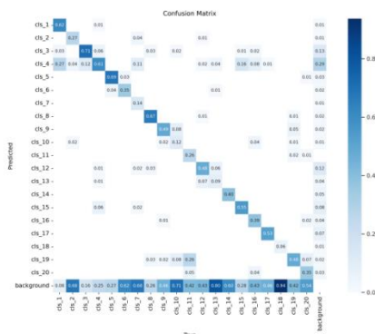
YOLOv5s
