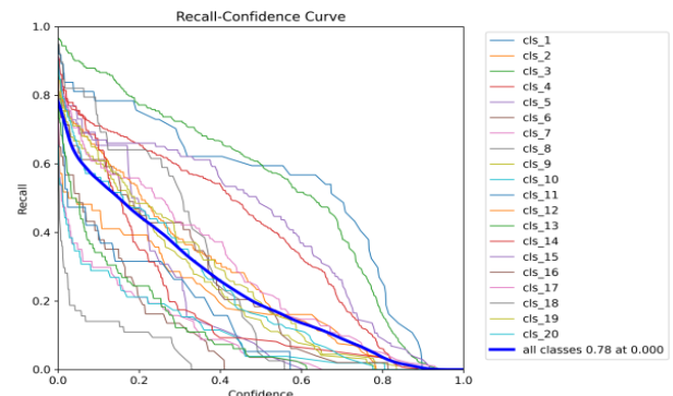
YOLOv5s-epsa
