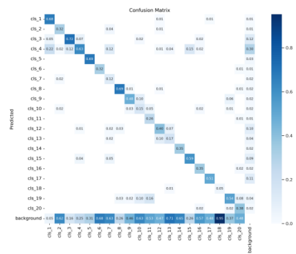
YOLOv5s-Bifpn
