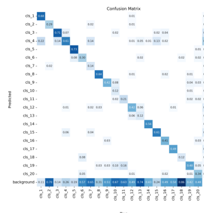
YOLOv5s-dcnv2
