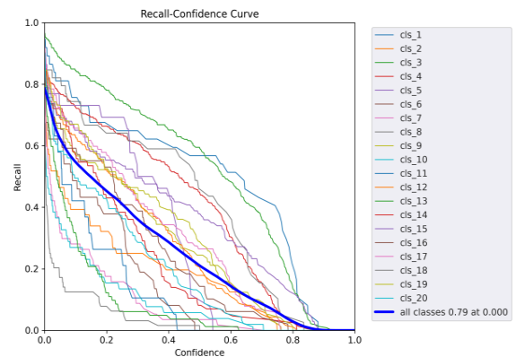
YOLOv5s-Bifpn
