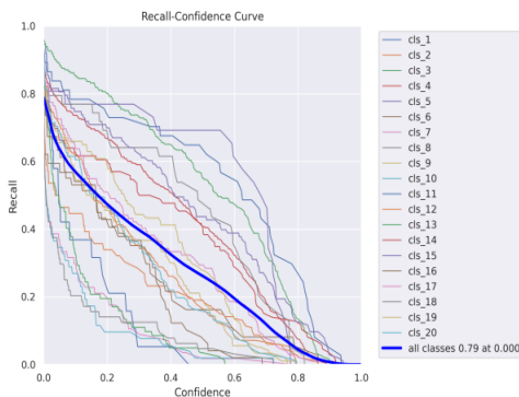
YOLOv5s-dcnv2
