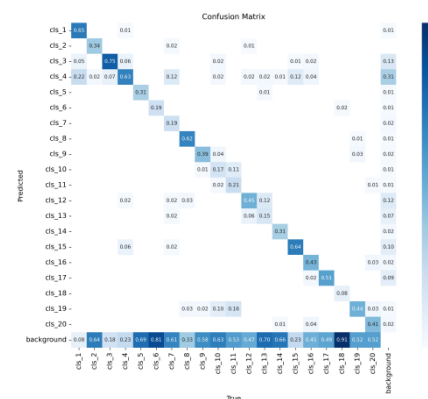
YOLOv5s-Bifpn
