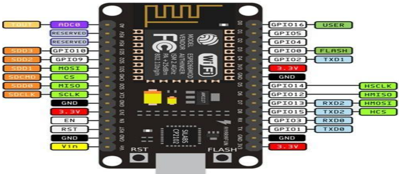
Fig. 2: ESP8266
