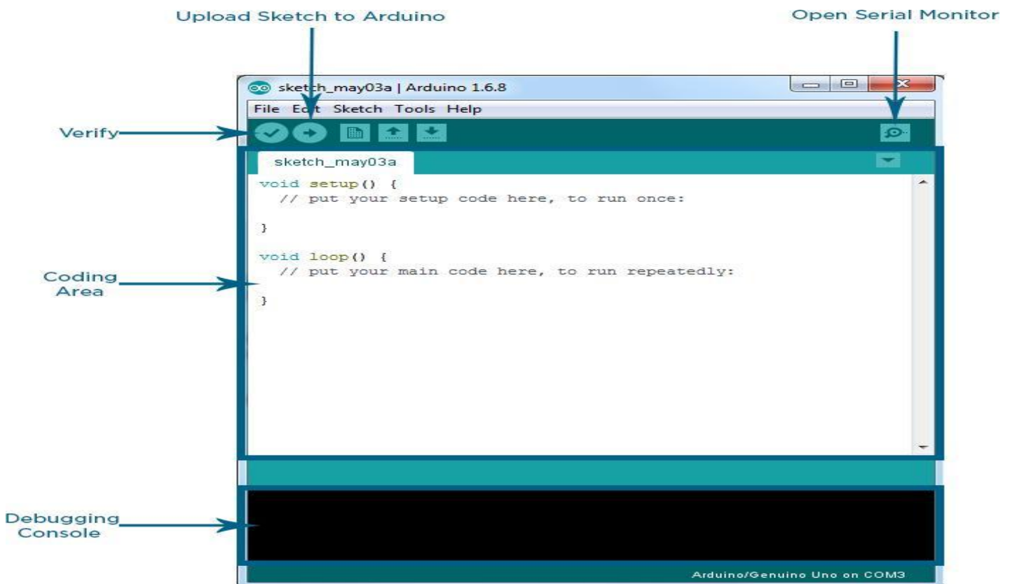
Fig. 7: Arduino IDE
