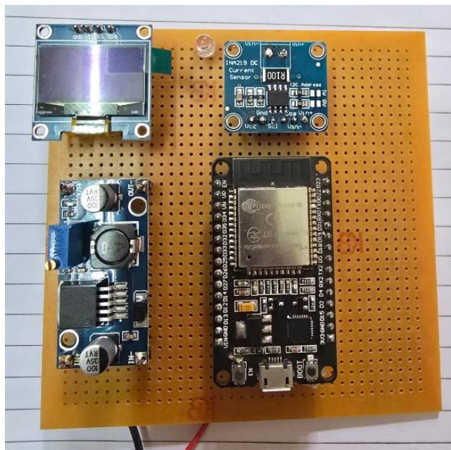
Figure 1. Actual Model
