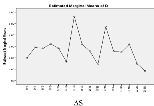
Fig 3: Estimated Marginal Means for (D)
